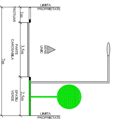
PROFIL TRANSVERSAL TIP PE STRADA CRINULUI 1
