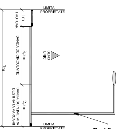
PROFIL TRANSVERSAL TIP PE STRADA CRINULUI 2
