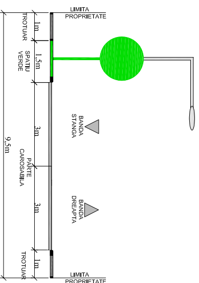
PROFIL TRANSVERSAL TIP PE STRADA CRINULUI 2
