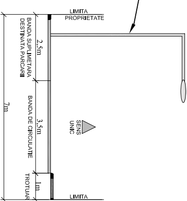
PROFIL TRANSVERSAL TIP PE STRADA CRINULUI 3
